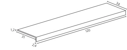
GRADINO PLUS** 34x120x4,5 cm Rect - 13 3/8 "x48"x1 3/4 " NATURALE ± 9,5 mm
